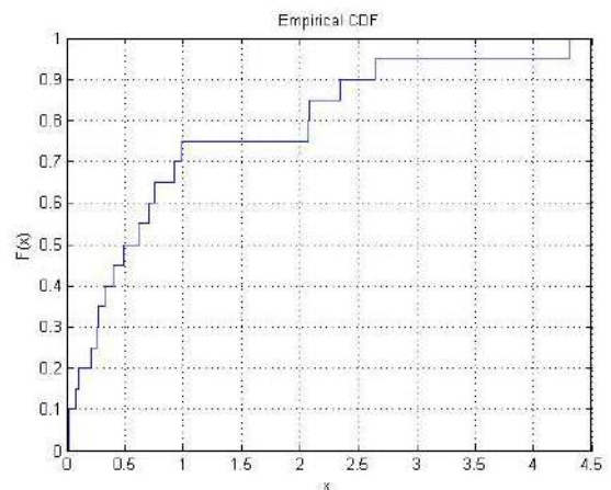
Рисунок 6 - Эмпирическая ФР
