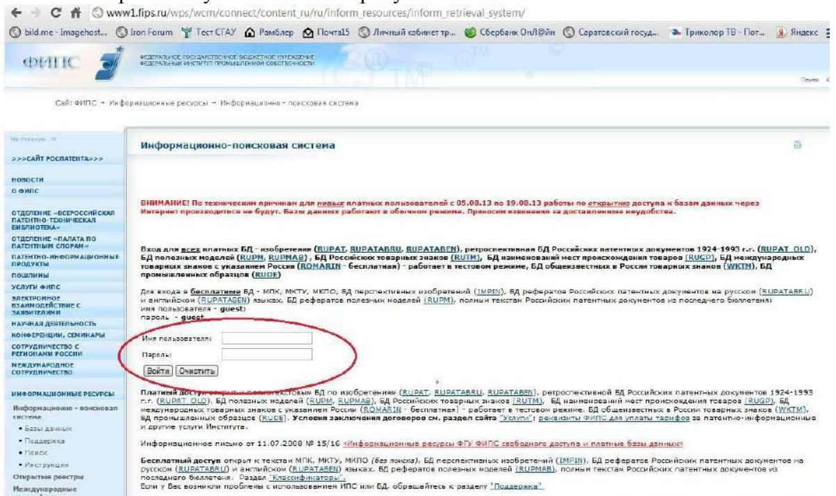
Рис. 4 Ввод пароля
