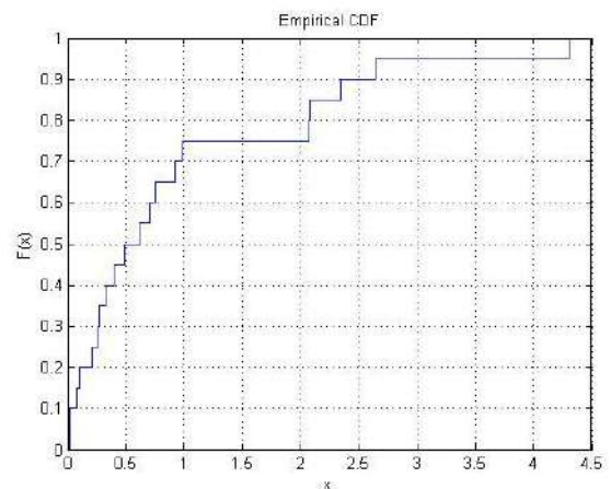
Рисунок 6 - Эмпирическая ФР
