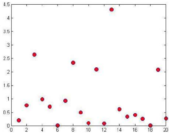
Рисунок 4 - Визуализация данных
