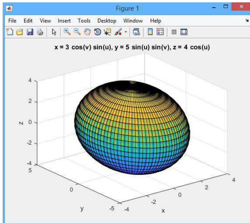
Рисунок 2 - Эллипсоид
