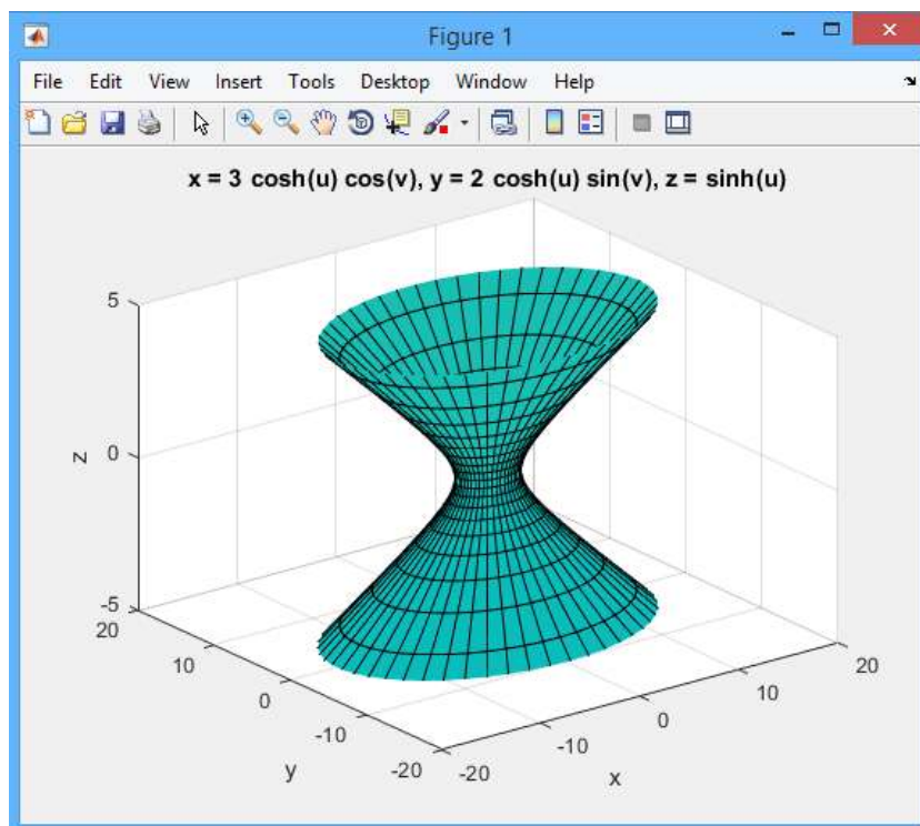
Рисунок 3 - Однополостный гиперболоид
